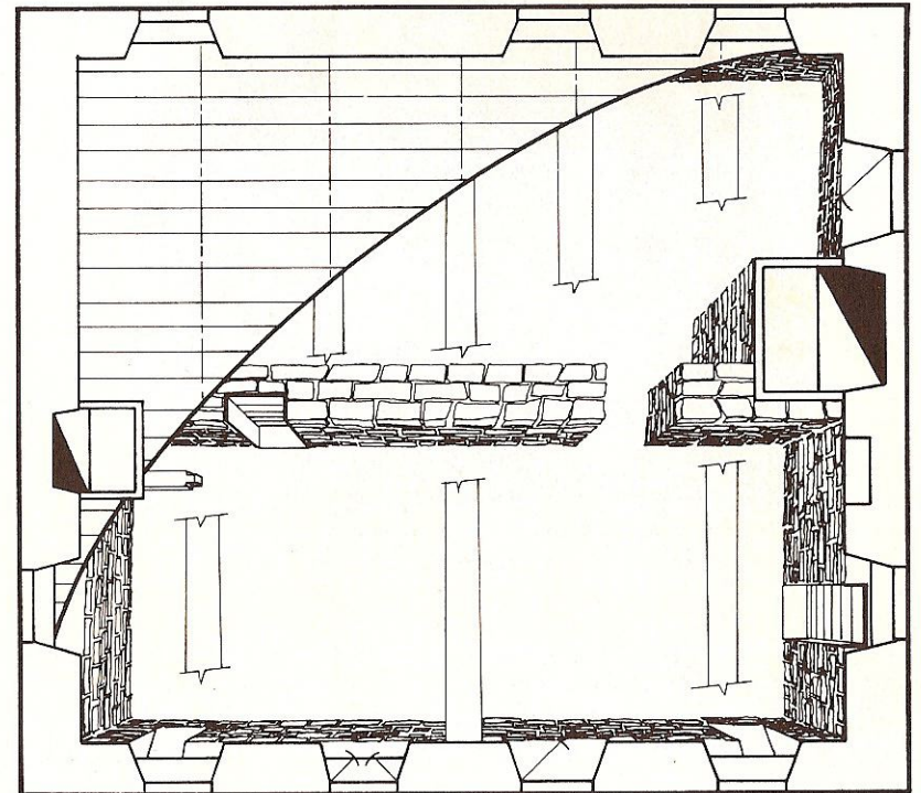
Coupe en plan du sous-sol et du rez-de-chaussée.
